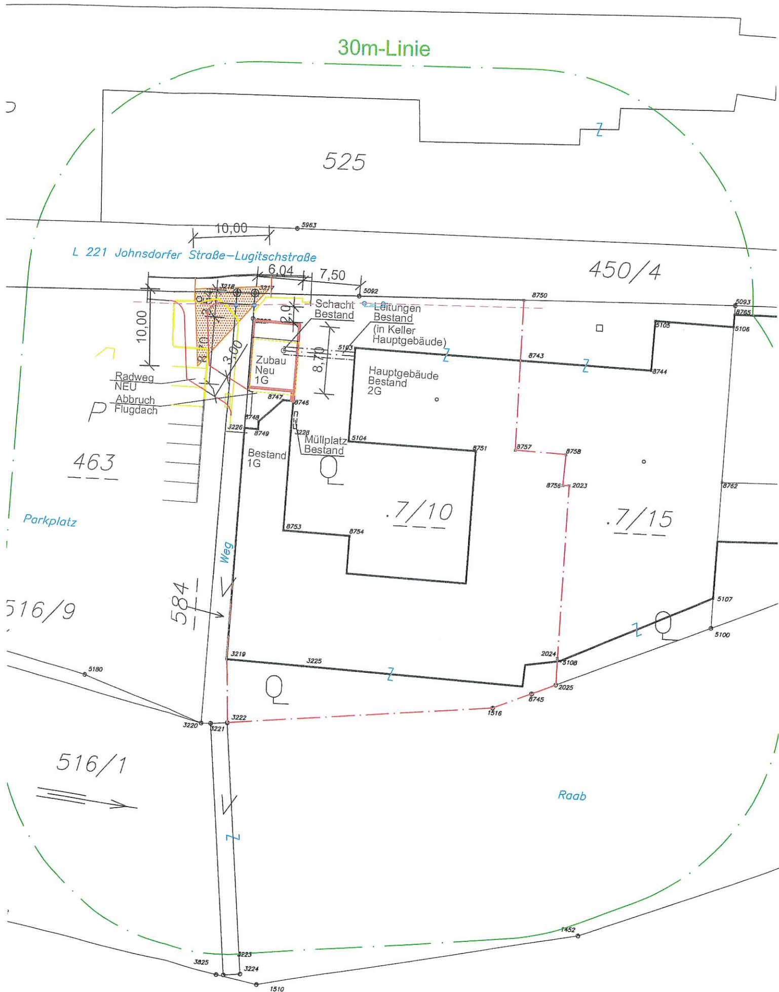
LAGEPLAN DKM
